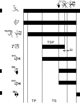
OPTIONS S e Snn
