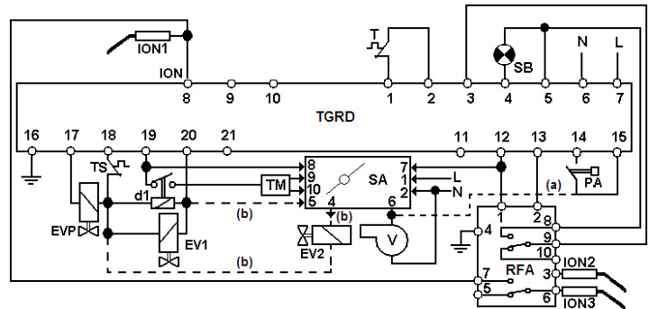
Type TGRD with option SA and RE3
