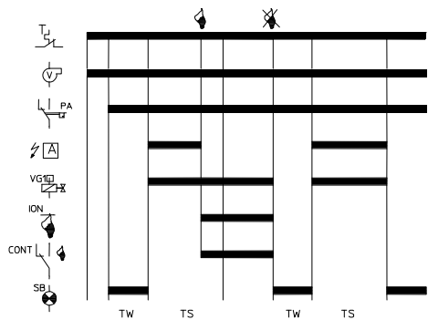
TYPE SE31F
