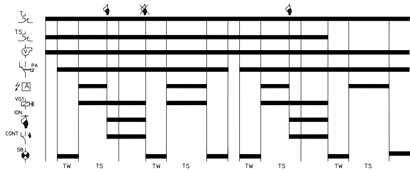
TYPE TE32F
