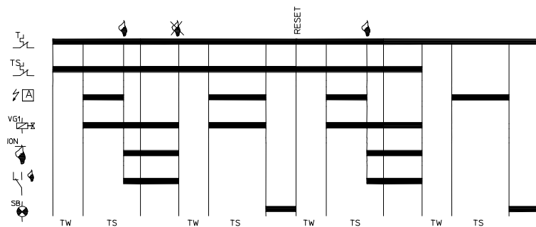
TYPE TM12F
