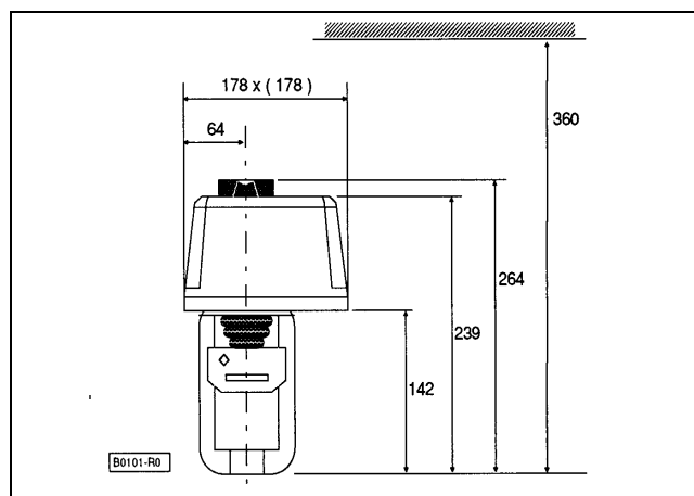
Fig. 2 M6421B/M7421B
