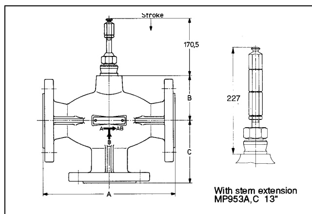
Fig. 1 V5015A
