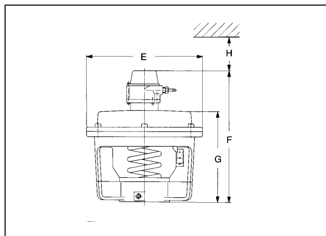
Fig. 3 MP953A,C
