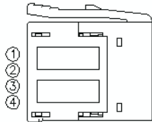
Y Connector pin layout
