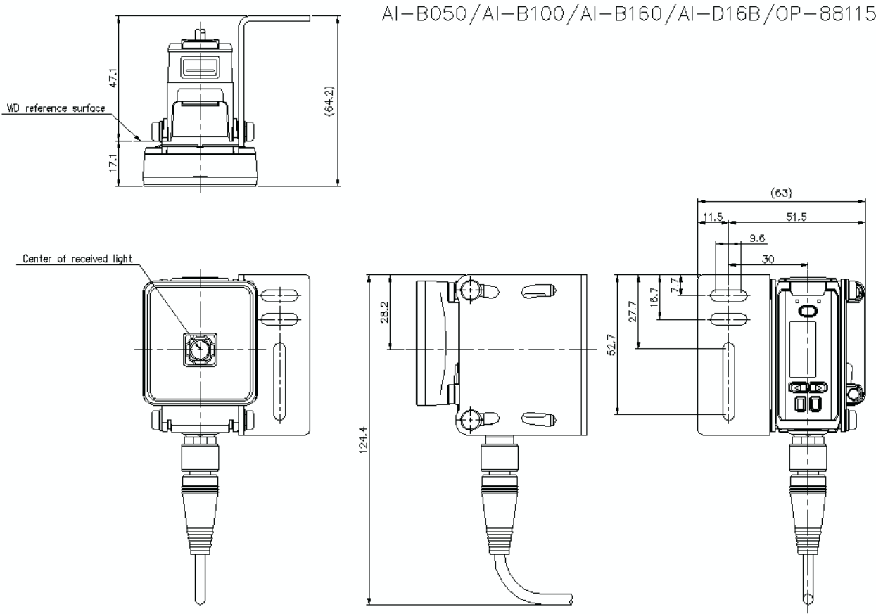
aib_d16b_88115_dimension_01.gif
