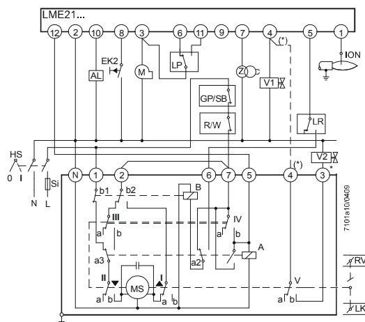
SQN3...121.../2-ступенчатое управление
