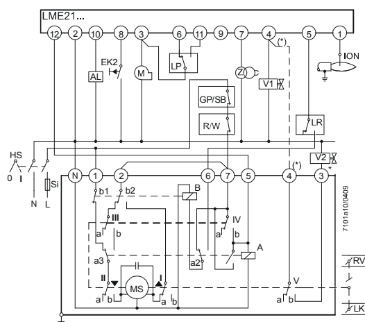
SQN3...121.../2-ступенчатое управление
