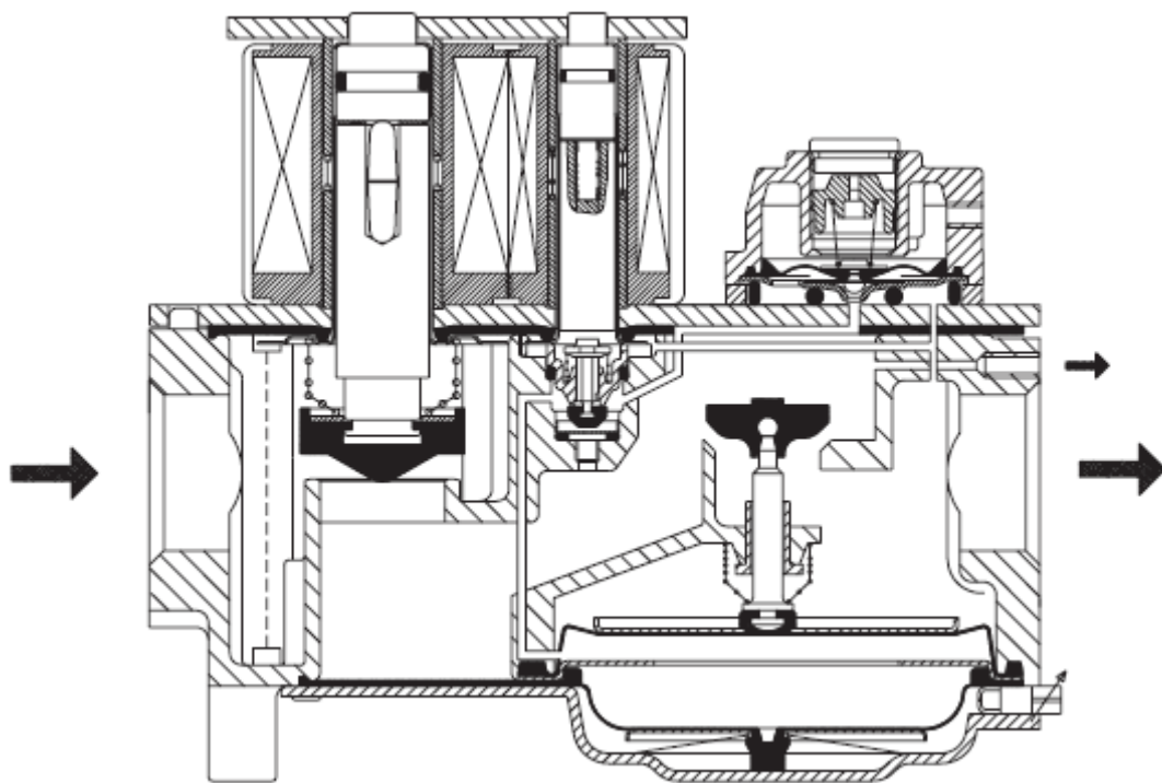
Рис. 14. Серворегулирование давления
