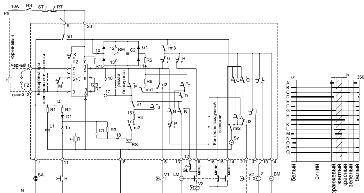
Электросхема ТМО 720-4
