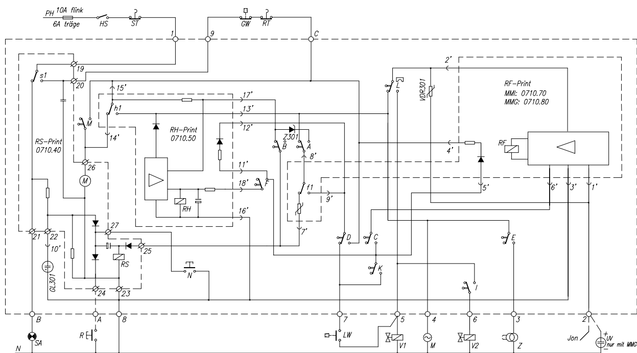
Электросхема MMI 811.1
