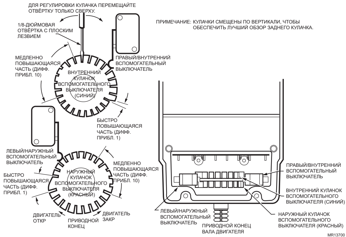
Рис. 14. Регулировка вспомогательных выключателей.
