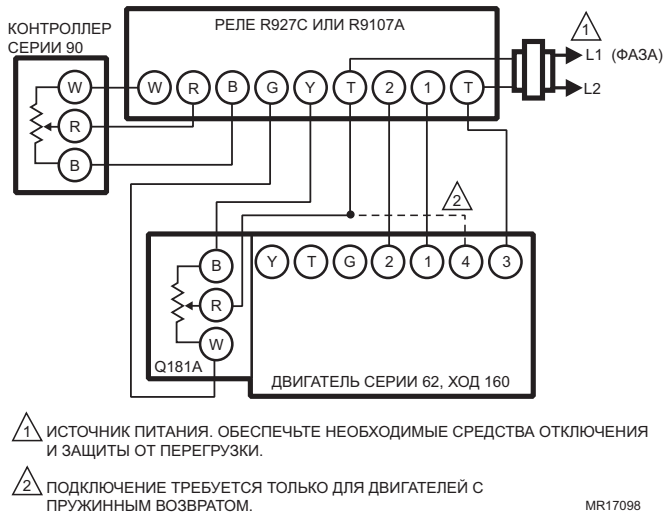
Рис. 8. Подключение через реле R927C или R9107A.
