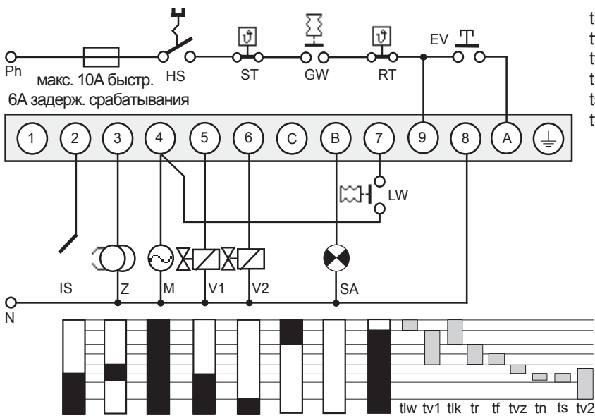
Схема соединений и диаграмма протекания программного цикла для DMG 973 без сервопривода воздушной заслонки
