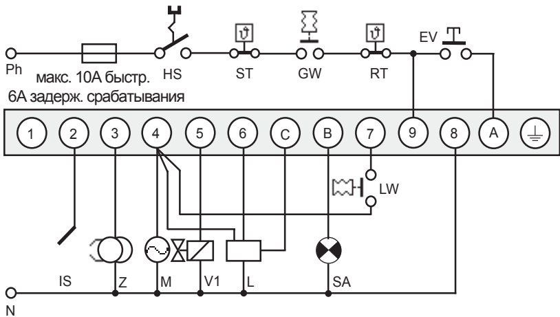
Схема соединений и диаграмма протекания программного цикла для DMG 973 без сервопривода воздушной заслонки
