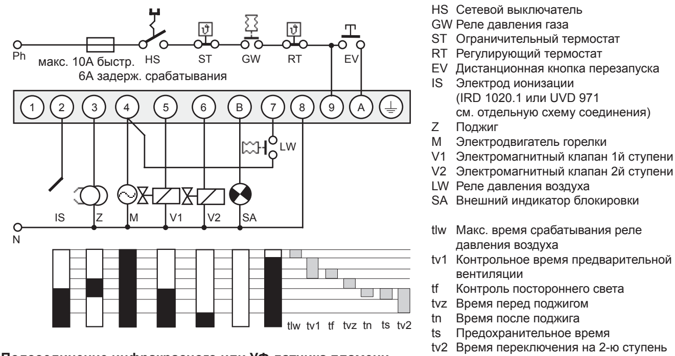
Подсоединение инфракрасного или УФ датчика пламени
