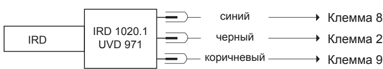
Подсоединение инфракрасного или УФ датчика пламени
