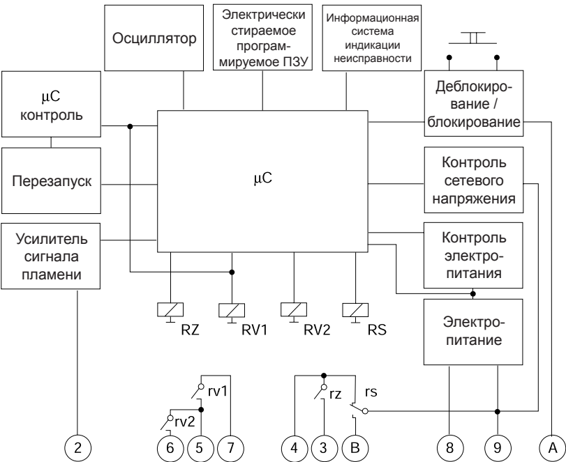
Блок-схема DMG 970
