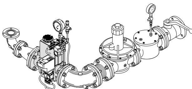
Линия низкого давления – фланцевая арматура с клапанами DMV без линии газа зажигания *
