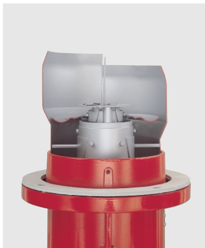
Подвижная пламенная труба устанавливается на горелку к теплогенератора в соответствии с типом теплогенератора и геометрий камеры сгорания
