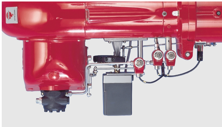
Регулирующий привод комбинированной горелки типа GL: газовая часть – плавно-двухступенчатое исполнение ZM, жидкотопливная часть – двухступенчатое
