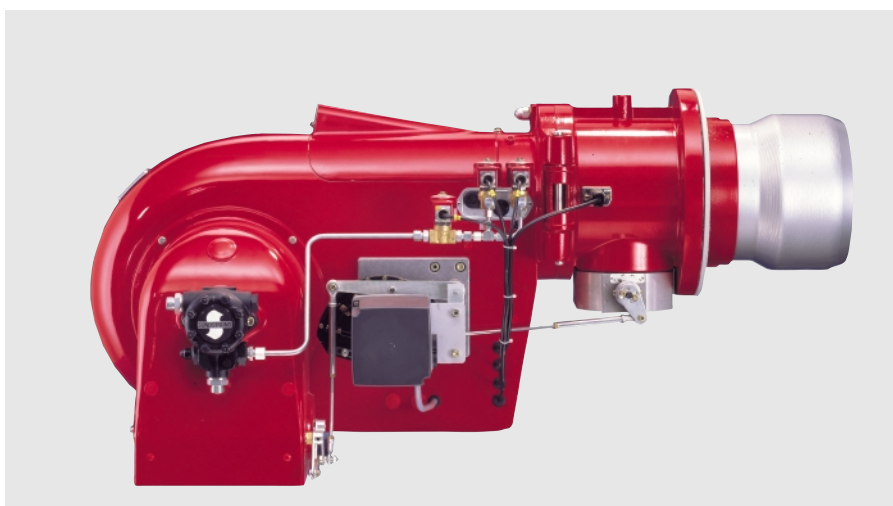
Комбинированная горелка типа GL, плавно-двухступенчатая (ZM) или модулируемая (M)
