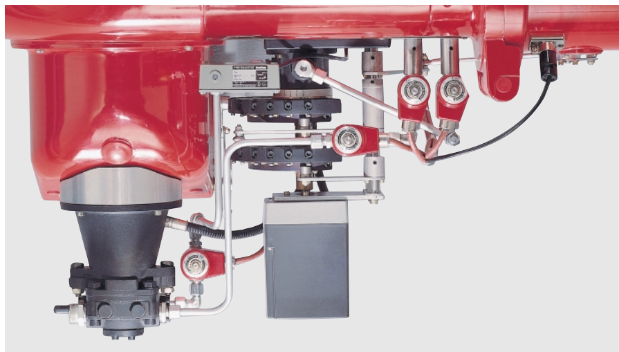
Регулирующий привод комбинированной горелки типа RGL: газовая и жидкотопливная часть – плавно-двухступенчатое исполнение ZM
