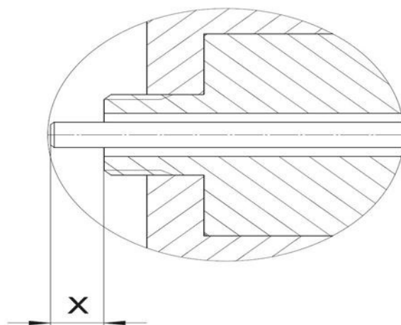
Fig. 56 X: расстояние (указательный шток)
