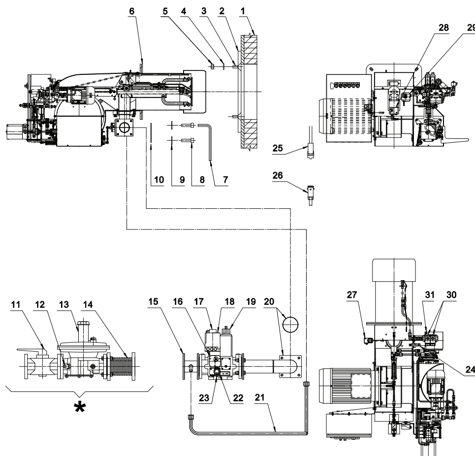
Fig. 4 УСТАНОВКА ГОРЕЛКИ
