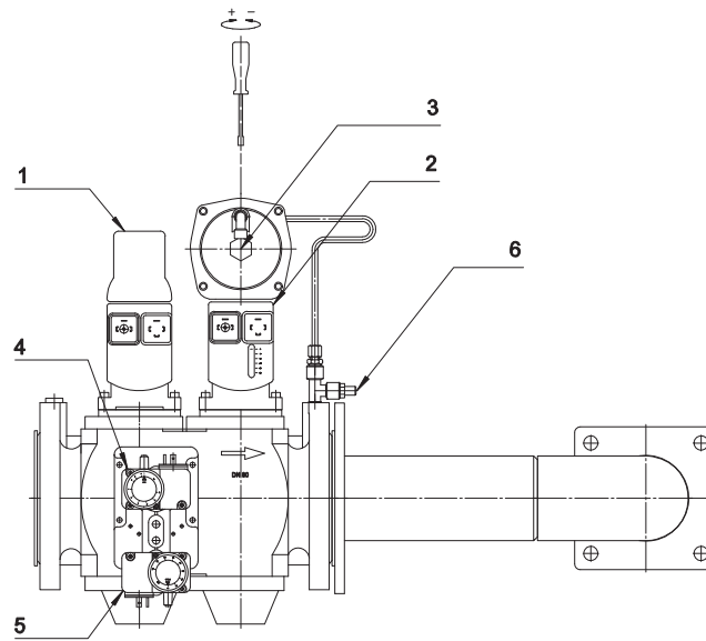
Fig. 22 ОСНОВНАЯ ГАЗОВАЯ РАМПА: SIEMENS VGD40...
