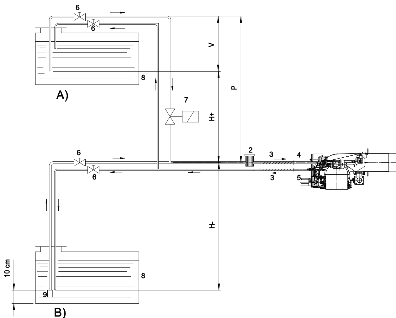
Fig. 11 гидравлического контура
