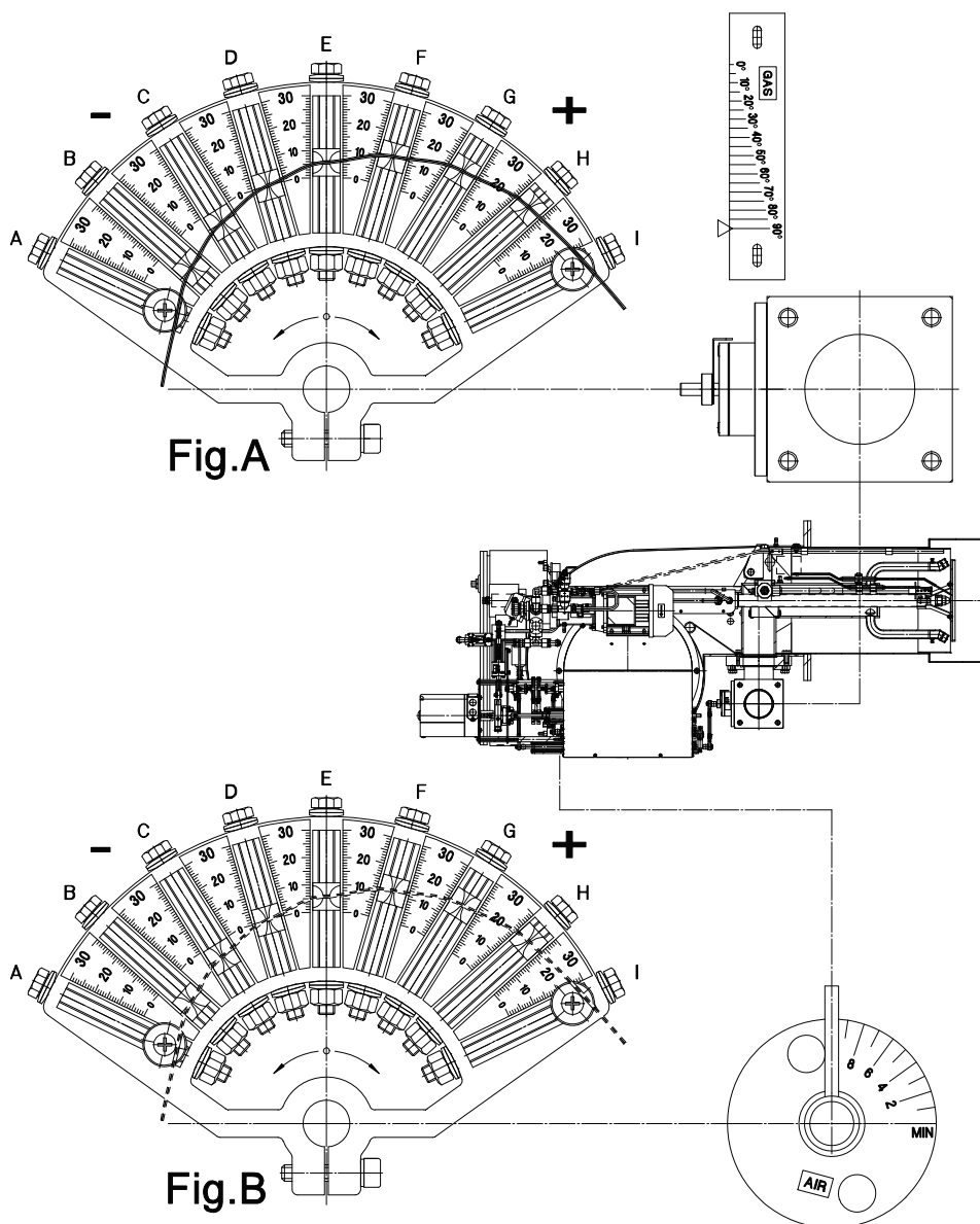
Fig. 33 НАСТРОЙКИ СЦЕНТРИКОВ К 190/М - К 250/М
