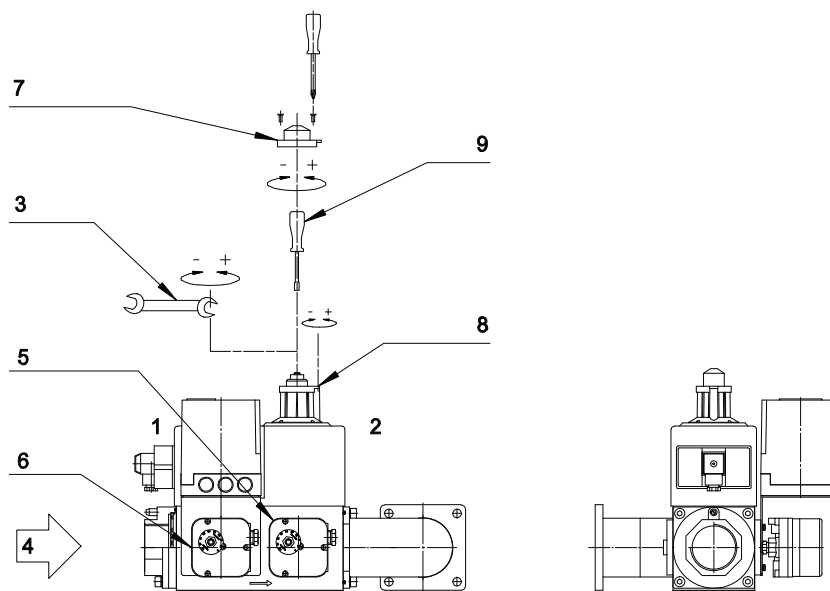
Fig. 19 ОСНОВНАЯ ГАЗОВАЯ РАМПА: HONEYWELL
