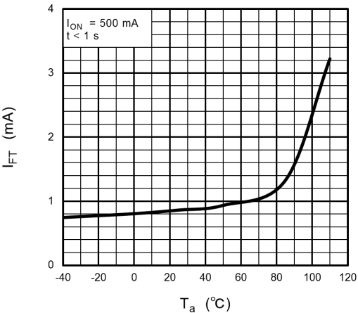
Fig. 14.1.6 I_{FT} - T_a
