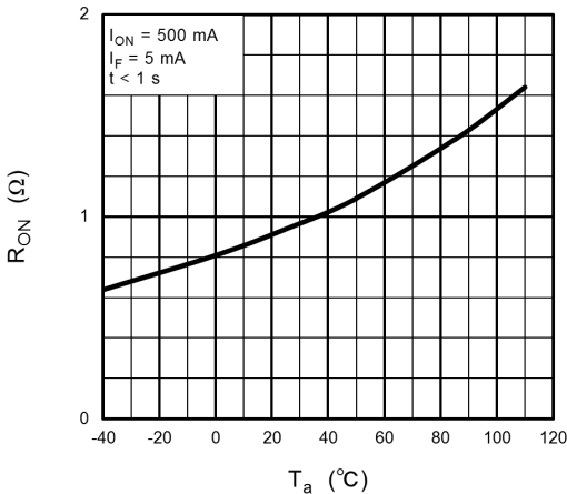
Fig. 14.1.5 R_{ON} - T_a
