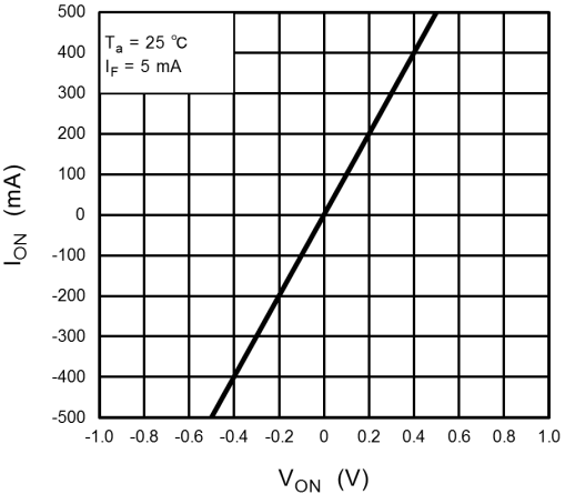
Fig. 14.1.4 I_{ON} - V_{ON}
