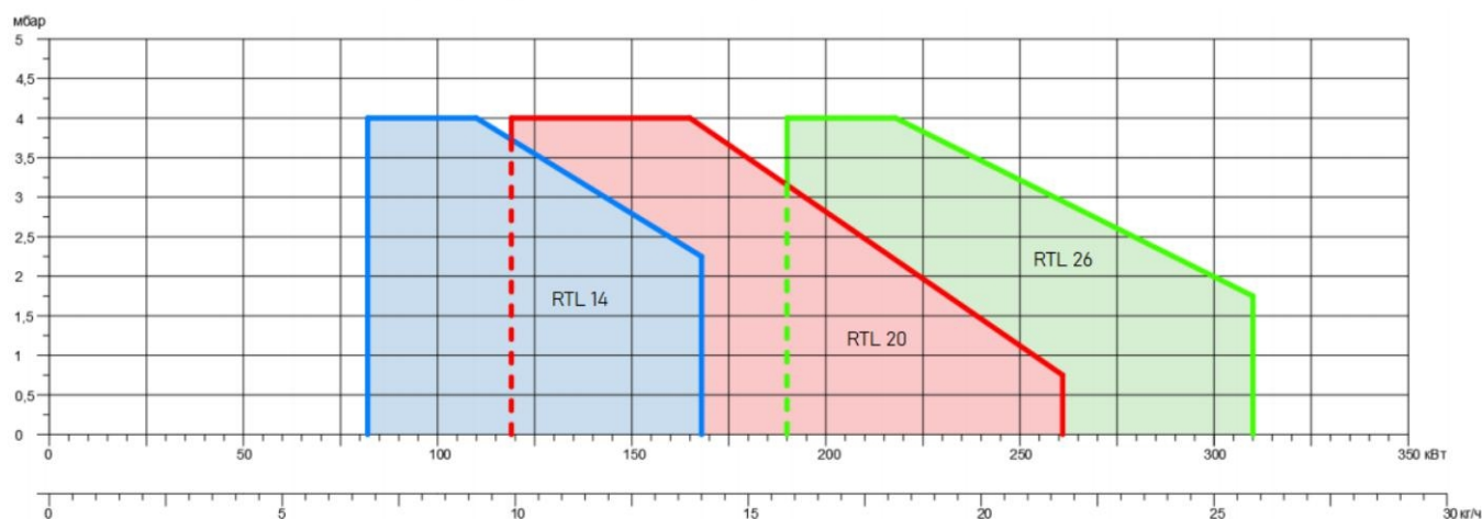
График рабочего поля горелок 14
