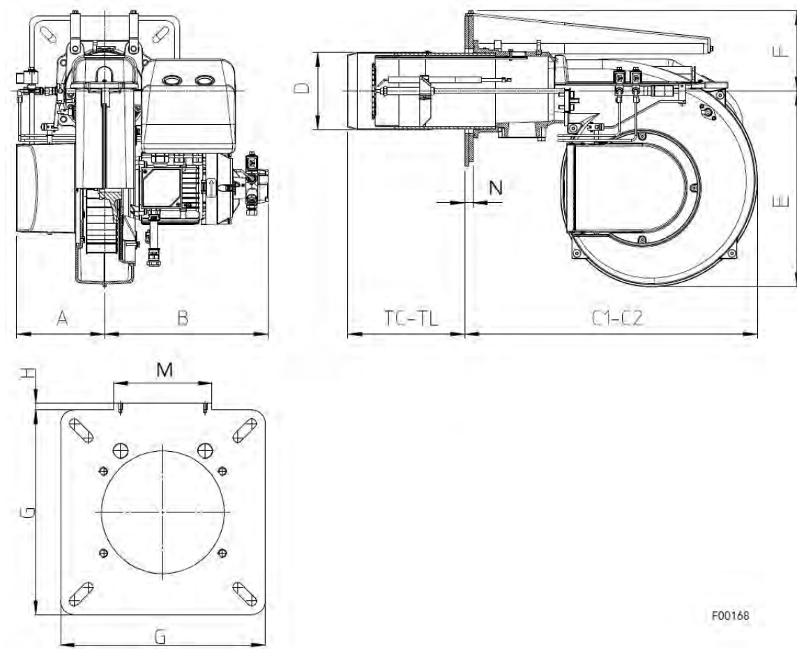
Fig. 5 РАЗМЕРЫ FGP 75/2
