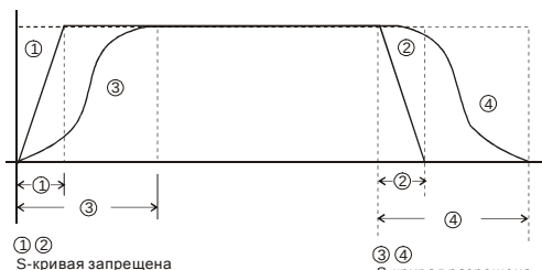
Характеристики разгона/торможения
