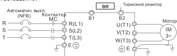
Схема 3 (для VFD-E-T, типоразмер A):
