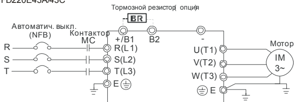
Схема 3 (для VFD-E-T, типоразмер A):
