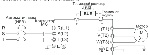
Схема 2 (для типоразмеров B): VFD007E11A, VFD015E21A, VFD022E21A/23A/43A VFD037E23A/43A, VFD007E11C, VFD015E21C, VFD022E21C/23C/43C, VFD037E23C/43C (для типоразмера C): VFD055E23A/43A, VFD075E23A/43A, VFD110E43A, VFD055E23C/43C, VFD075E23C/43C, VFD110E43C (для типоразмера D): VFD150E23A/23C, VFD150E43A/43C, VFD185E43A/43C, VFD220E43A/43C
