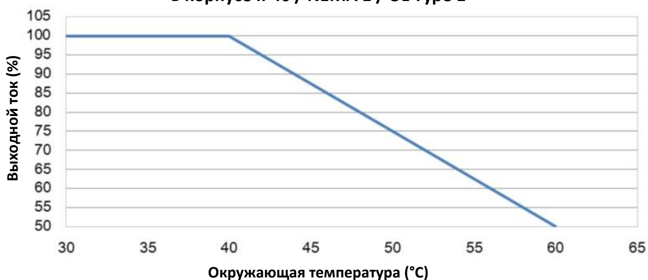
Снижение характеристик в зависимости от температуры окружающей среды в корпусе IP40 / NEMA 1 / UL Type 1
