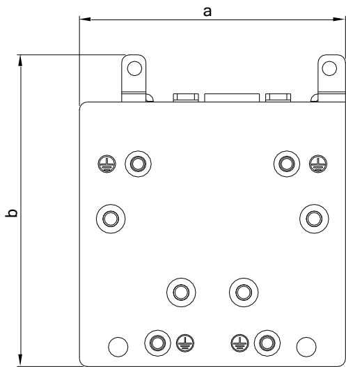
Размеры панели крепления экранов
