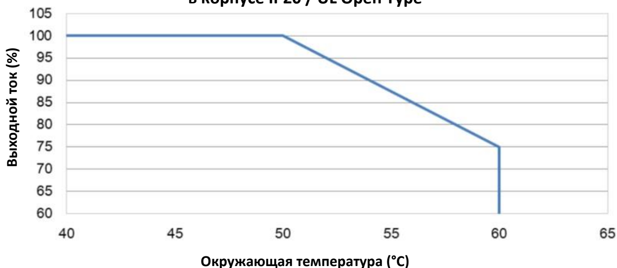
Снижение характеристик в зависимости от температуры окружающей среды в корпусе IP20 / UL Open Type
