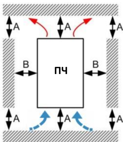
Установка одиночного преобразователя
