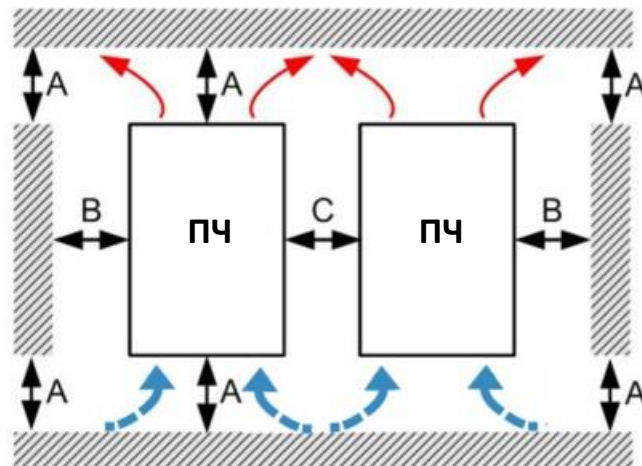
Горизонтальная установка сторона к стороне
