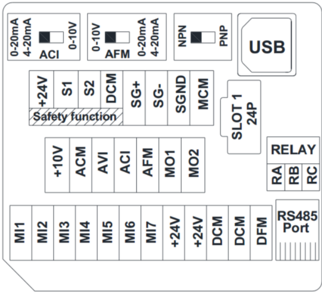
Расположение клемм управления
