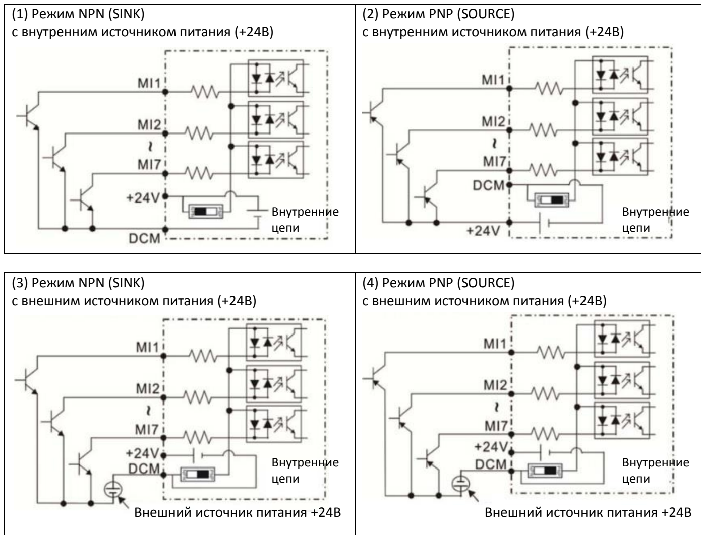
Рисунок 2 Варианты подключения NPN / PNP
