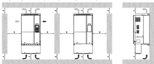
Рис. 4. Несколько ПЧ: Плотная установка (типоразмеры А-С)
