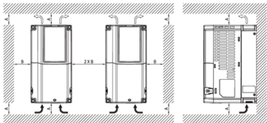
Рис. 3. Несколько ПЧ: Установка без взаимовлияния с перегородкой (типоразмеры D-E)
