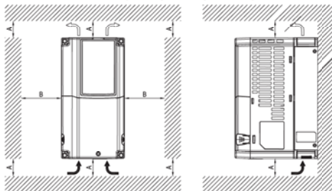
Рис. 1. Один ПЧ (типоразмеры А-Е)
