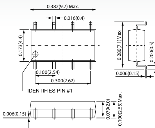
C334S
