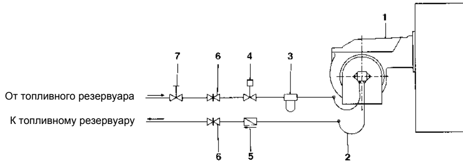
Рис. 11 - Двухтрубная система
