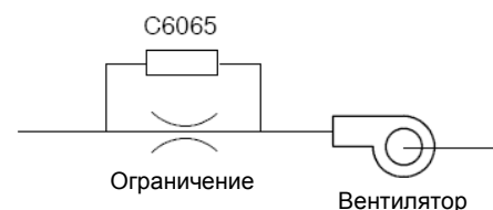
Рис. 2. Схема воздушного тракта
