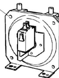
Рис. 10. Общий вид реле С6065
