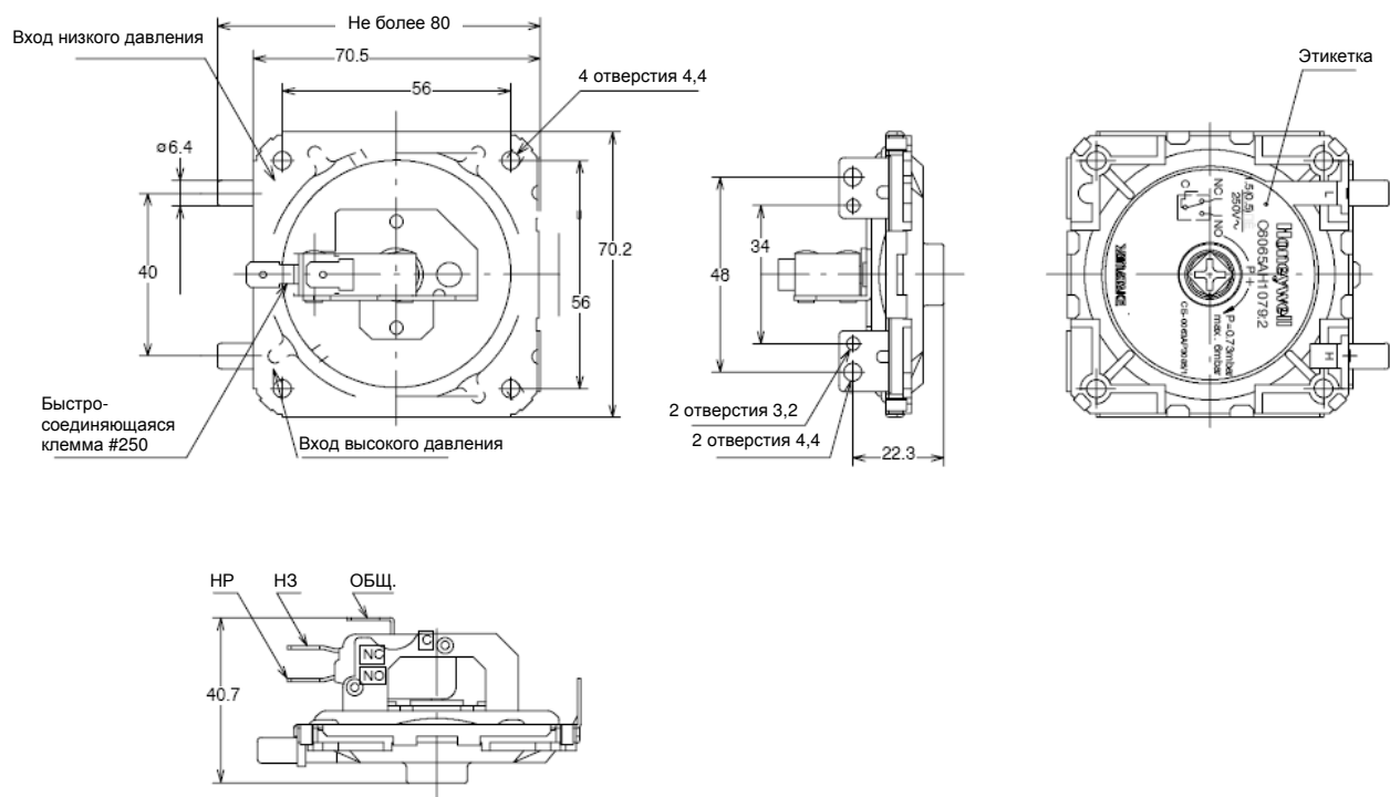
Рис. 5. Чертежи с размерами
