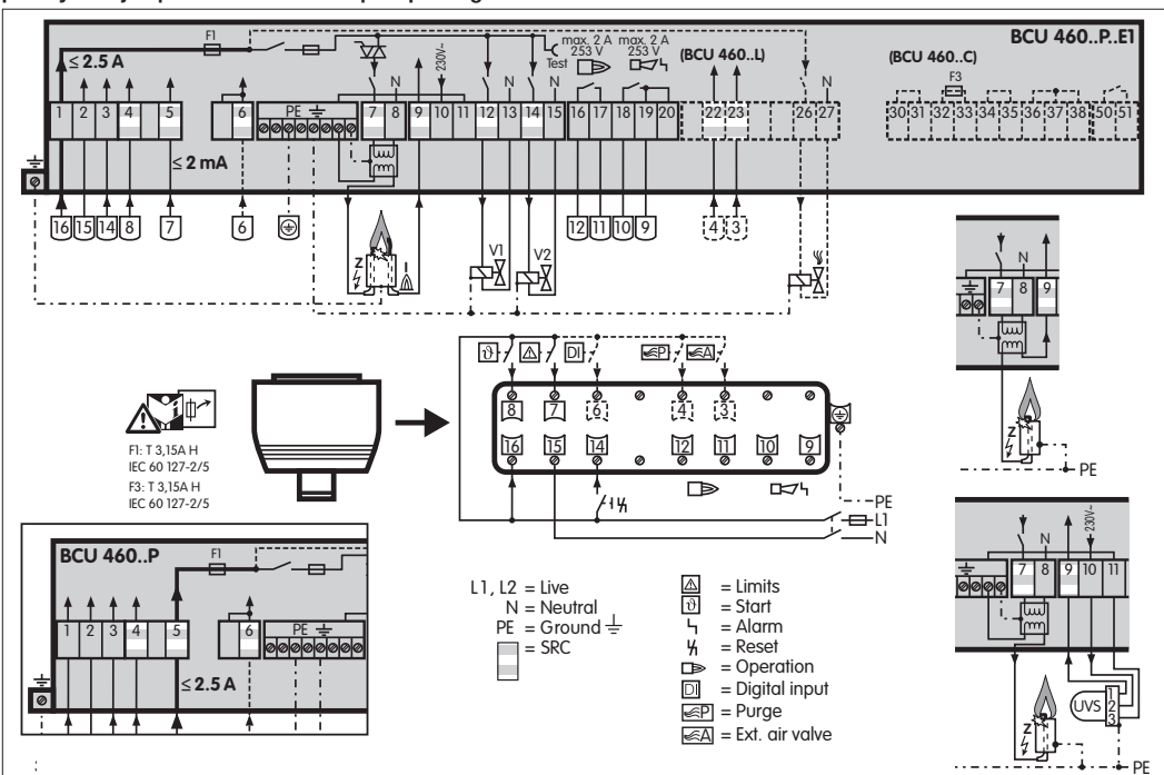
BCU 460..P..E1, BCU 460..P mit Industriestecker/Sanayi tipi soket ile/s průmyslovou zástrčkou/z wtyczką wg normy przemysłowej/с промышленным штекером/ipari dugasszal
