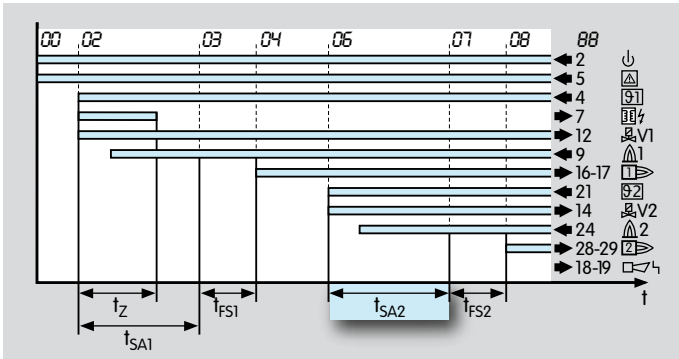
Время безопасности t_{SA2} для основной горелки при запуске
