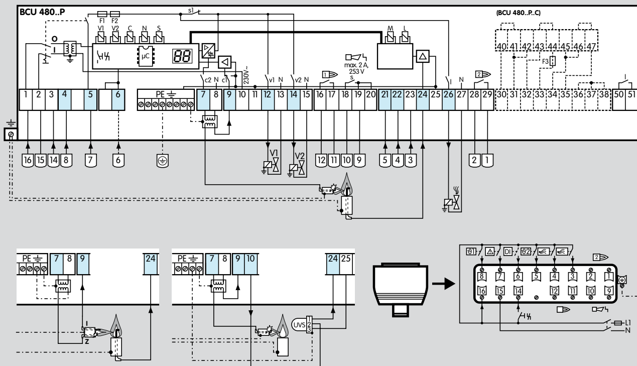
BCU 480..P с промышленным штекером Обозначения на схеме - смотри Обозначения.
