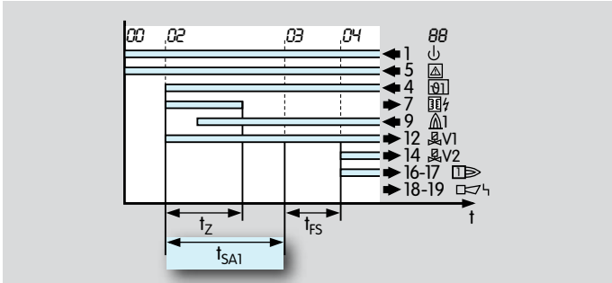
Время безопасности t_{SA1} для пилотной горелки при запуске
