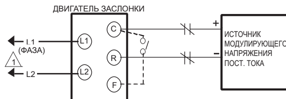
Рис. 5. Типичная система электропроводки.
