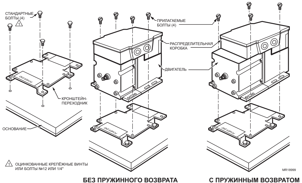
Рис. 3. Монтаж двигателя с использованием кронштейна-переходника.
