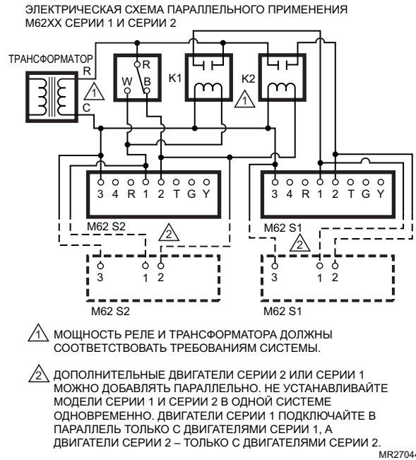
Рис. 9. Параллельное применение двигателей серии 1 и серии 2.
