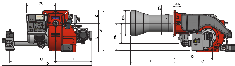
DN65 - DN80
