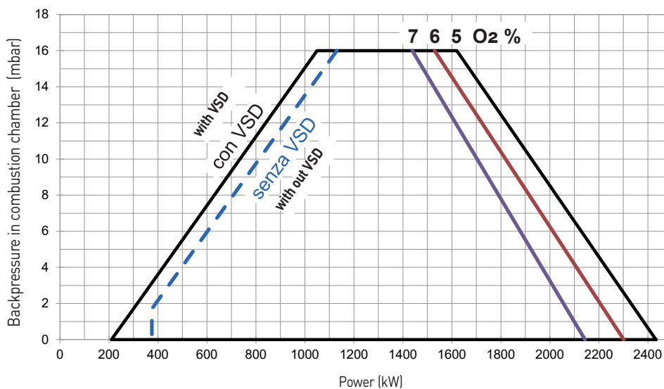
G240N PR-MD
