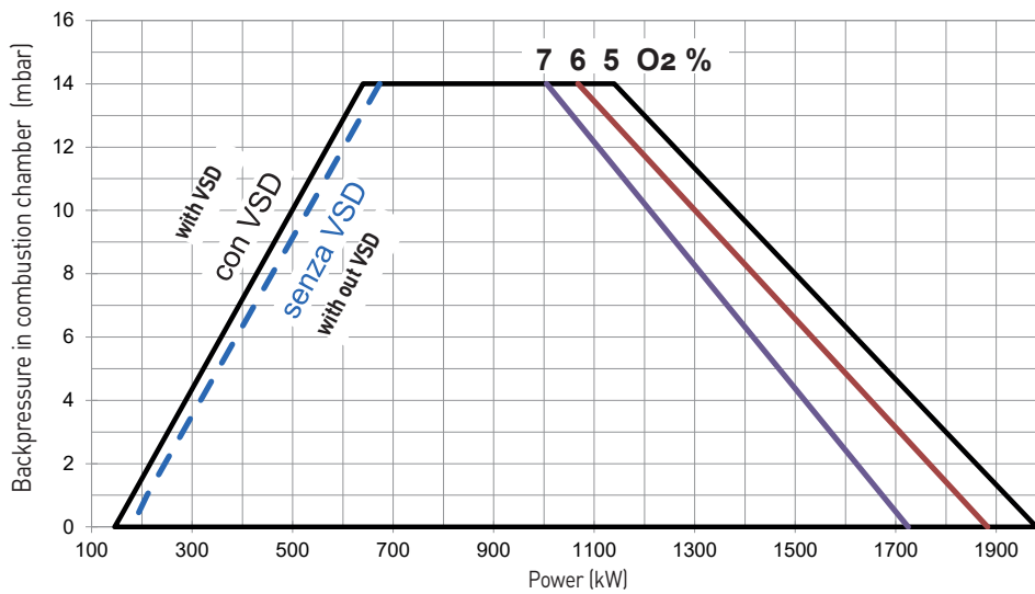
G200N PR-MD
